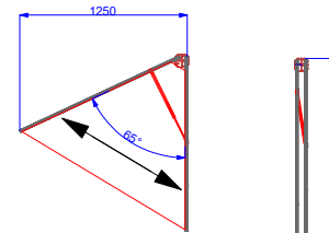
JiffyJoy 132/125/65° Balkon mit Geländer Din rechts
