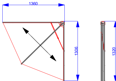
JiffyJoy 136/132/90° Balkon mit Geländer Din rechts
